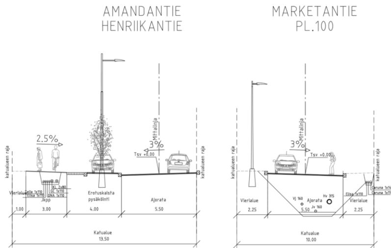
Amadantien ja Henriikantien tyypipoikkileikkaus ja Marketantien tyypipoikkileikkaus. Kuva: WSP Finland Oy
