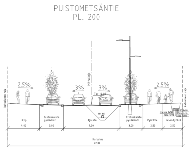
Kokoojakadun tyypipoikkileikkaus (Puistometsäntie), Kuva: WSP Finland Oy
